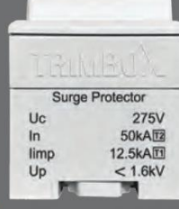
B+C Sınıfı 2 Kutuplu Parafudr (50kA) YM1T1T2
