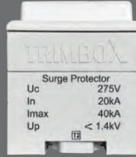
C Sınıfı 4 Kutuplu Parafudr (20/40kA) YM3T2
