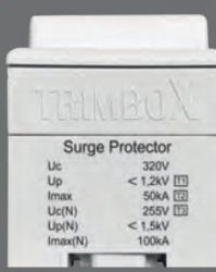
B+C+D Sınıfı 4 Kutuplu 100kA Parafudr YM4T1T2T3
