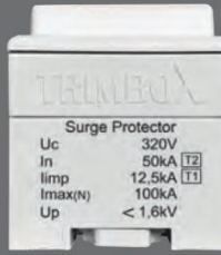
B+C Sınıfı 2 Kutuplu 100 kA Parafudr YM2T1T2
